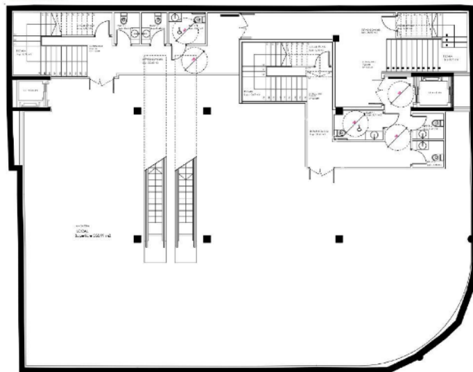
Planta soterrani
