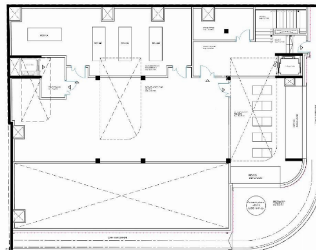
Segona planta
