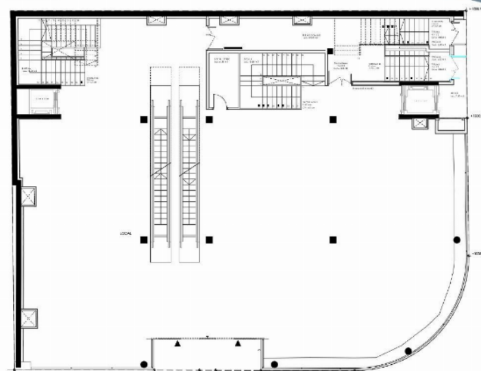
Planta baixa
