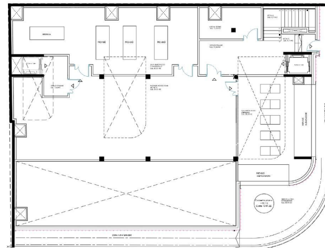
Primera planta
