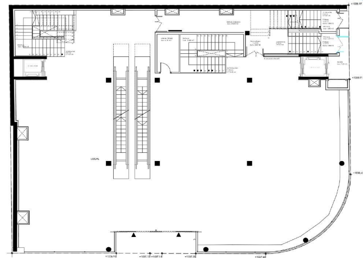
Planta baixa
