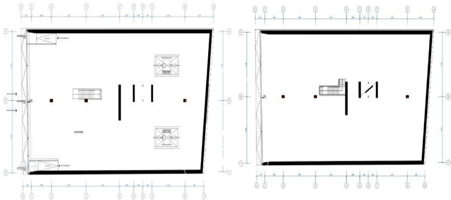
Planta +1
