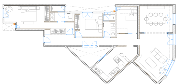
Plano Propuesta
