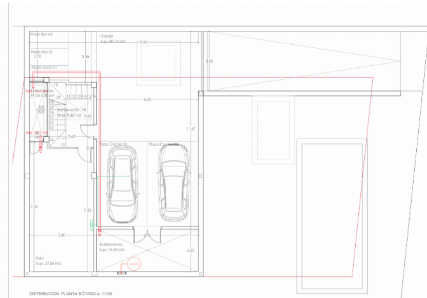
DISTRIBUCIÓN PLANTA SÓTANO a. 1/100
