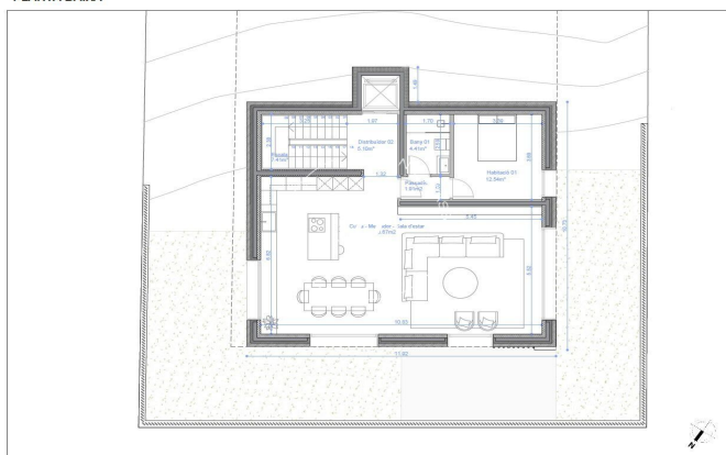
PROPOSTA PLANTA BAIXA
