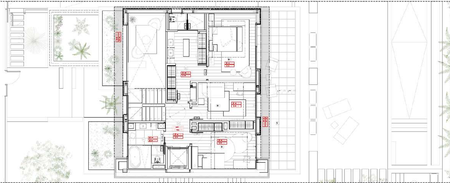
PLANTA BAJA - DISTRIBUCIÓN Y SUPERFICIES
