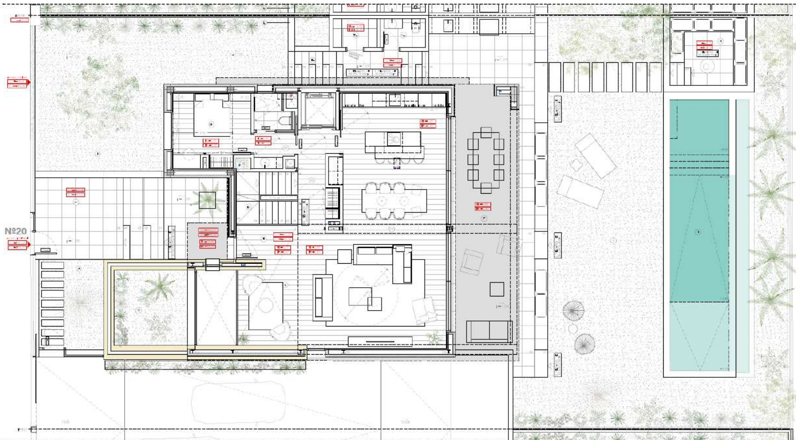
PLANTA BAJA - DISTRIBUCIÓN Y SUPERFICIES
