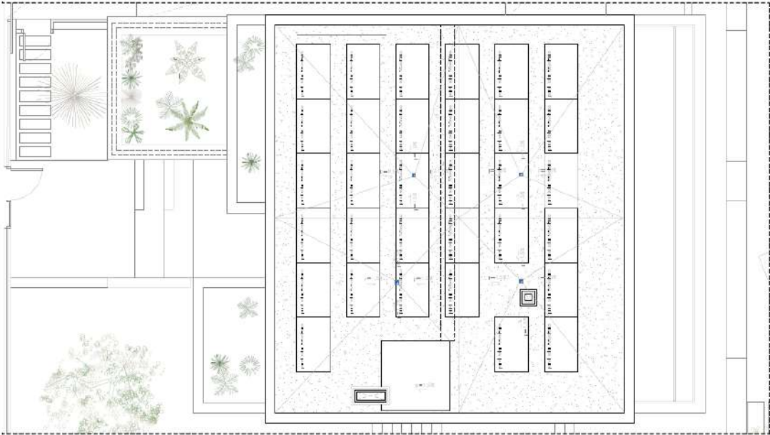
PLANTA CUBIERTA - DISTRIBUCIÓN Y SUPERFICIES
