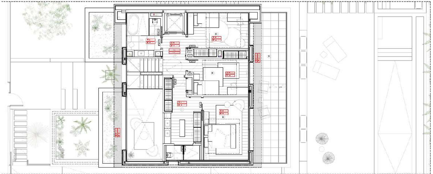
PLANTA BAJA - DISTRIBUCIÓN Y SUPERFICIES
