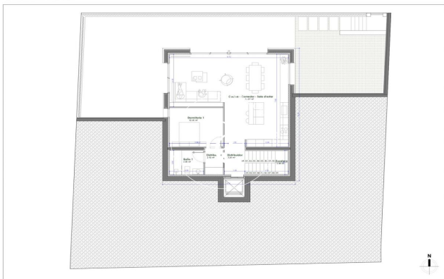
PROPOSICIÓN PRIMERA PLANTA
